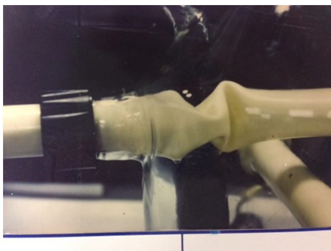
Foto 1 Een door toluene in de dampfase verweekte PVC buis.
